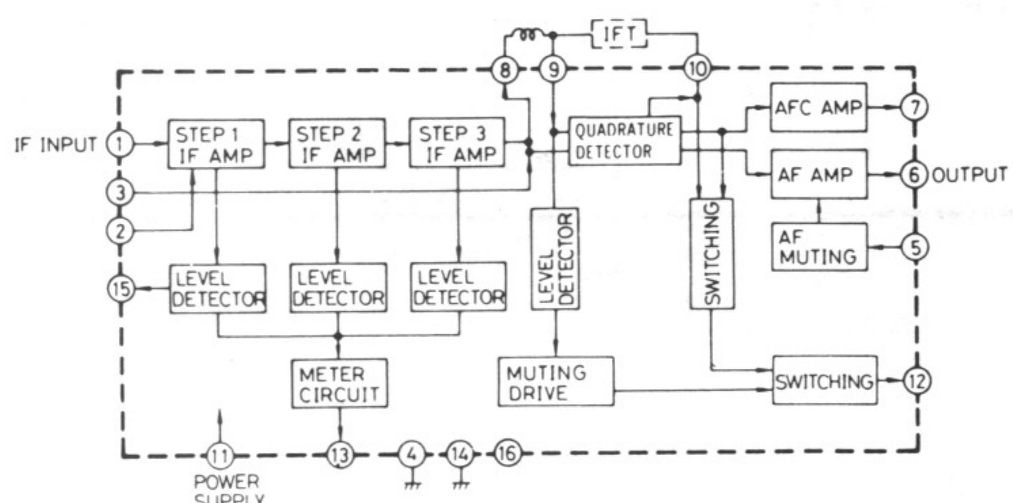
IC102 (AN377) FM IF Amplifier & Detector
